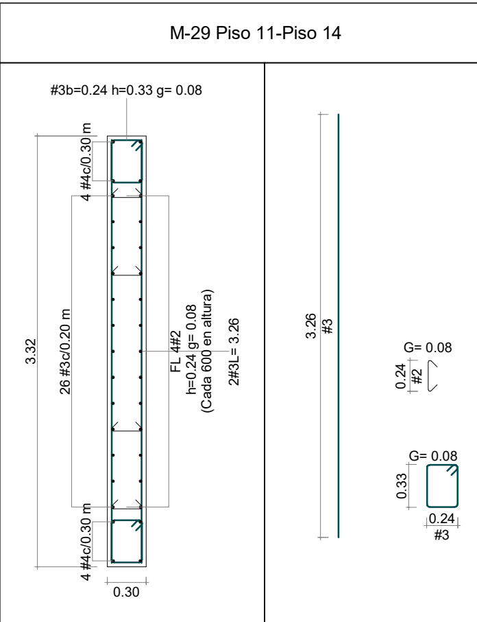
DETALLE SOBRE ANCHO EN MURO M-29
