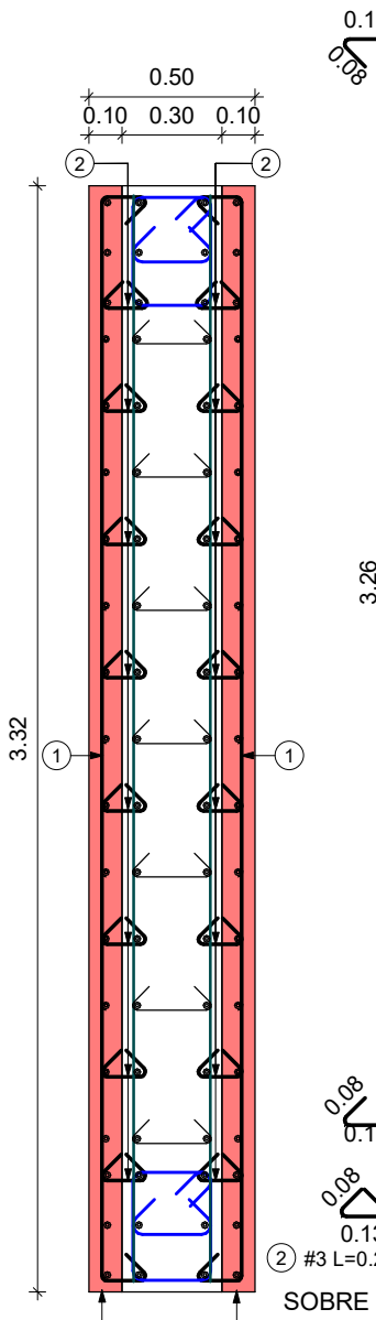
DETALLE SOBRE ANCHO EN MURO M-29
